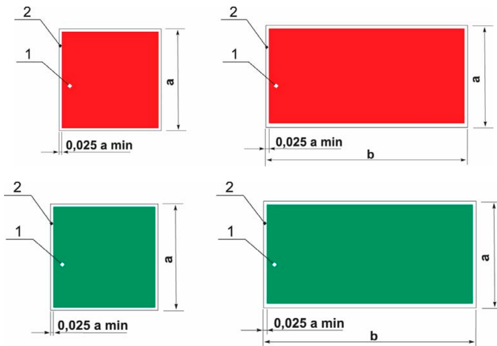
Рисунок 4 – Основа цветографического изображения и соотношение размеров указательных знаков пожарной безопасности
