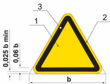
Рисунок 2 – Основа цветографического изображения и соотношение размеров предупреждающих знаков пожарной безопасности
